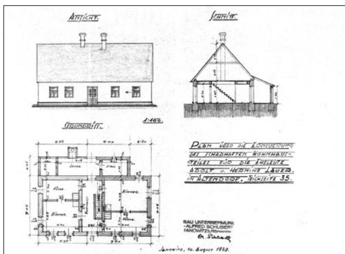
Plán renovace poškozené části obytného domu pro manžele Adolfa a Hermine Lauerovy ze Staré Vsi, 1939
