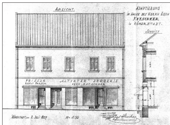
Adaptace v domě Egona Kutschkera v Rýmařově – náhled, řez, 1937
