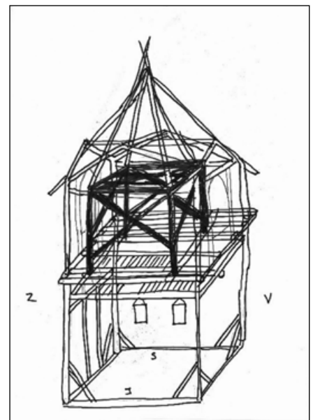
Náčrt zvonice s vestavěnou konstrukcí zvonové stolice (vyznačena tmavě)
