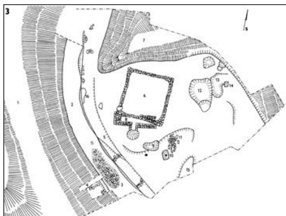
8. Hrádek na konci 13. stol., zařízení tavičské dílny (palác 6, vyhřívací zařízení 8, dílna 16, sklad rudy 12, pražírna 13)
