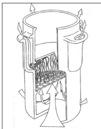
9B. Funkce uvedené pícky S. Matighofera z Č. Budějovic ze 16. století (systém M. Ernée, 2001)
