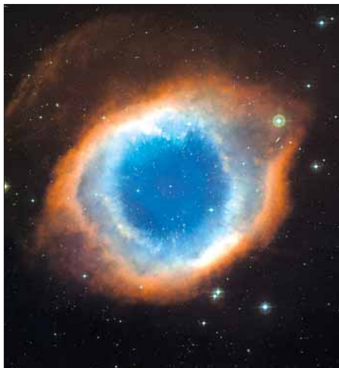
Helix - planetární mlhovina s bílým trpaslíkem uprostřed
